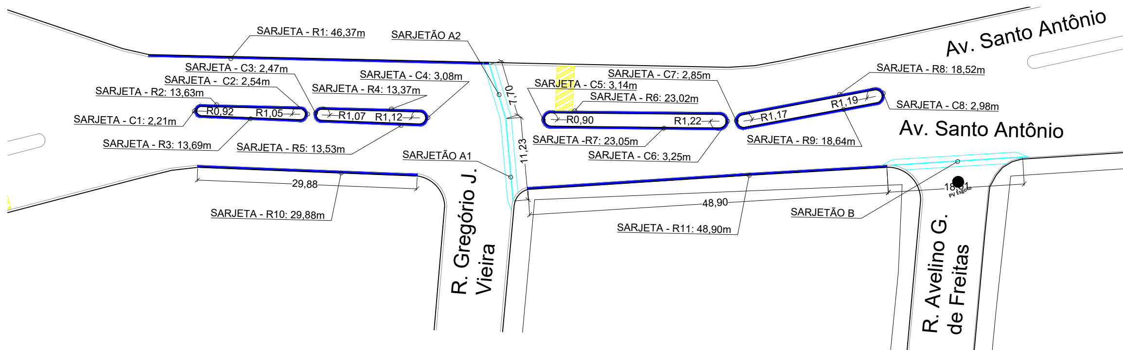
PROJETO DE CANALETAS (SARJETÃO) E SARJETAS - AVENIDA SANTO ANTONIO ESCALA 1:500
