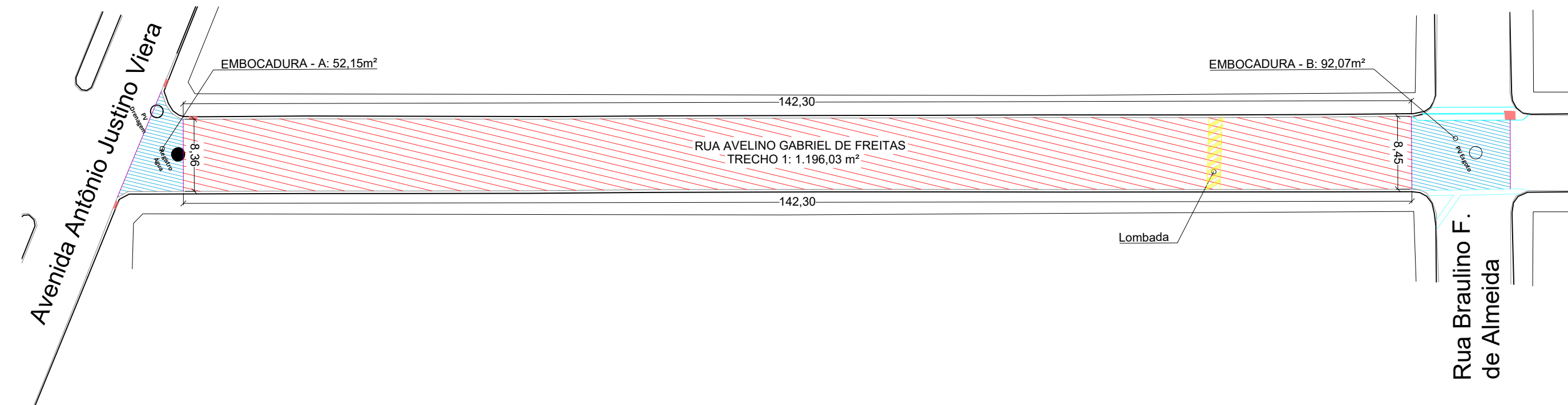
PROJETO DE RECAPEAMENTO EM CBUQ - RUA AVELINO GABRIEL DE FREITAS ESCALA 1:500
