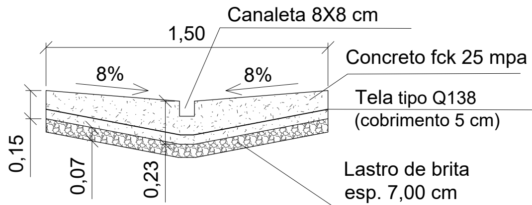
DETALHE - CANAleta (SARJETÃO) ESCALA 1:20
