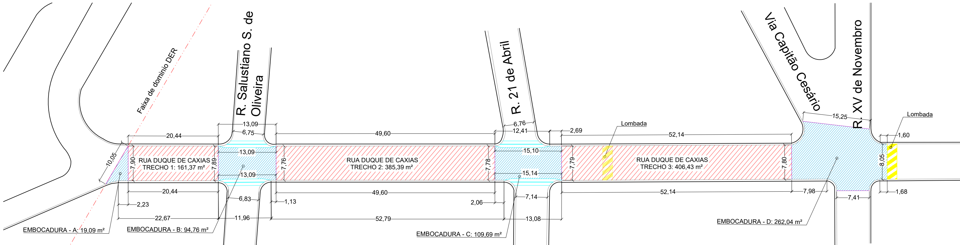
PROJETO DE RECAPEAMENTO EM CBUQ - RUA DUQUE DE CAXIAS ESCALA 1:500
