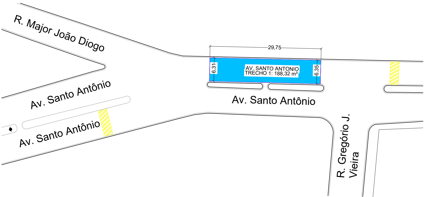
PROJETO DE RECONSTRUÇÃO DE BASE - AVENIDA SANTO ANTONIO ESCALA 1:500
