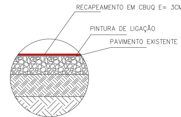
DETALHE DO RECAPEAMENTO EM CBUQ SEM ESCALA
