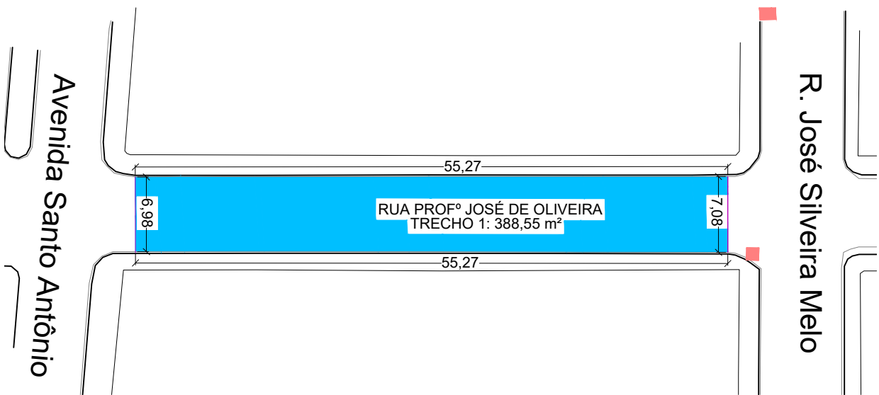
PROJETO DE RECONSTRUÇÃO DE BASE - RUA PROFESSOR JOSÉ DE OLIVEIRA ESCALA 1:500
