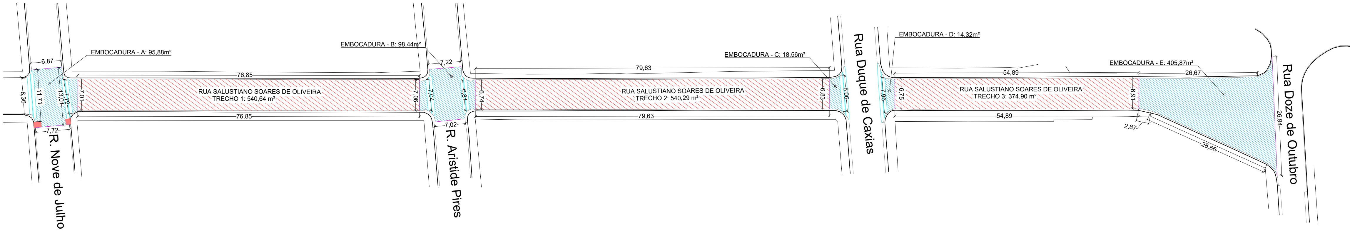
PROJETO DE RECAPEAMENTO EM CBUQ - RUA SALUSTIANO SOARES DE OLIVEIRA ESCALA 1:500
