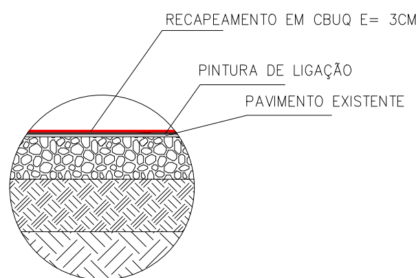
DETALHE DO RECAPEAMENTO EM CBUQ SEM ESCALA
