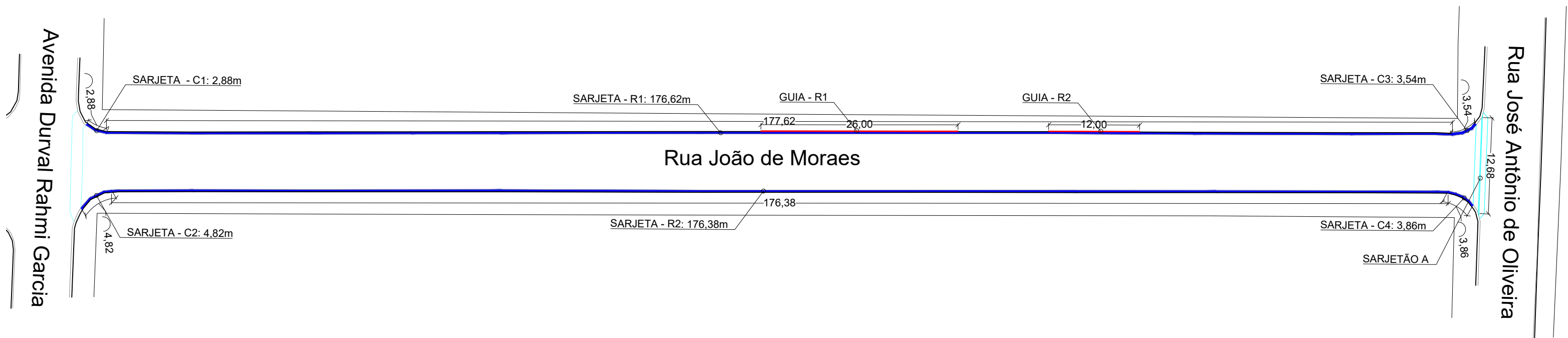
PROJETO DE CANALETAS (SARJETÃO), GUIAS E SARJETAS - RUA JOÃO DE MORAES ESCALA 1:500
