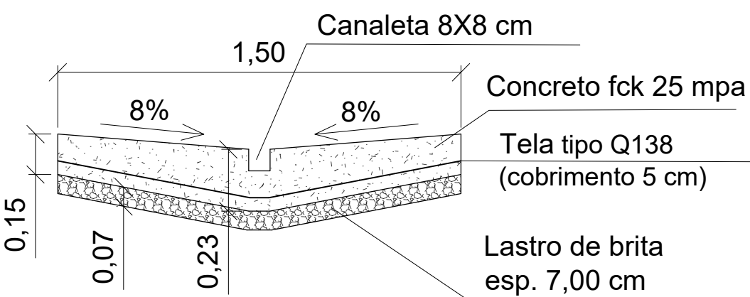
DETALHE - CANALETA (SARJETÃO) ESCALA 1:20
