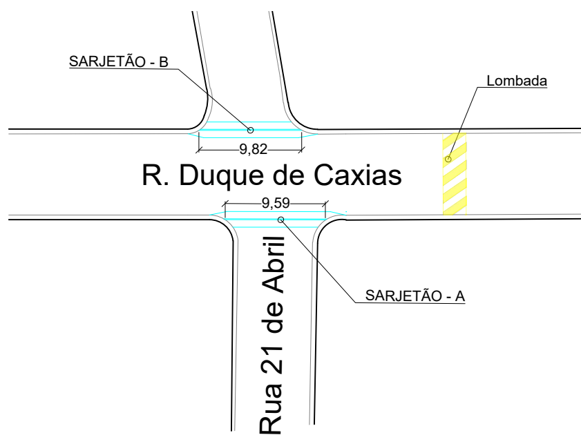
PROJETO DE CANALETAS (SARJETÃO) - RUA DUQUE DE CAXIAS ESCALA 1:500
