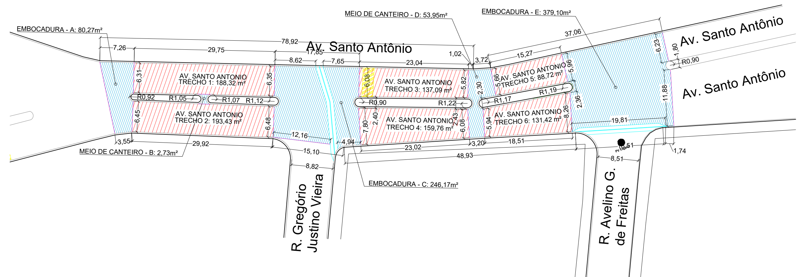
PROJETO DE RECAPEAMENTO EM CBUQ - AVENIDA SANTO ANTÔNIO ESCALA 1:500
