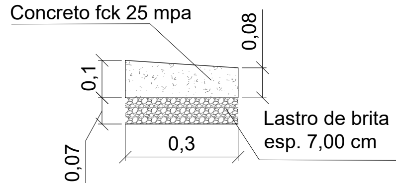
DETALHE DO SARJETA ESCALA 1:10
