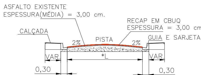
SEÇÃO TRANSVERSAL (GENÉRICA) - RECAPEAMENTO SEM ESCALA
