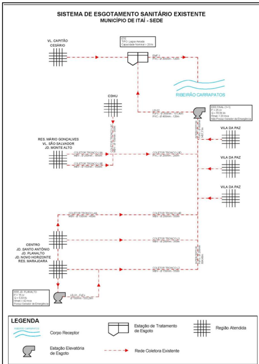
Figura 2 – Croqui do sistema de esgotamento de Itaí
