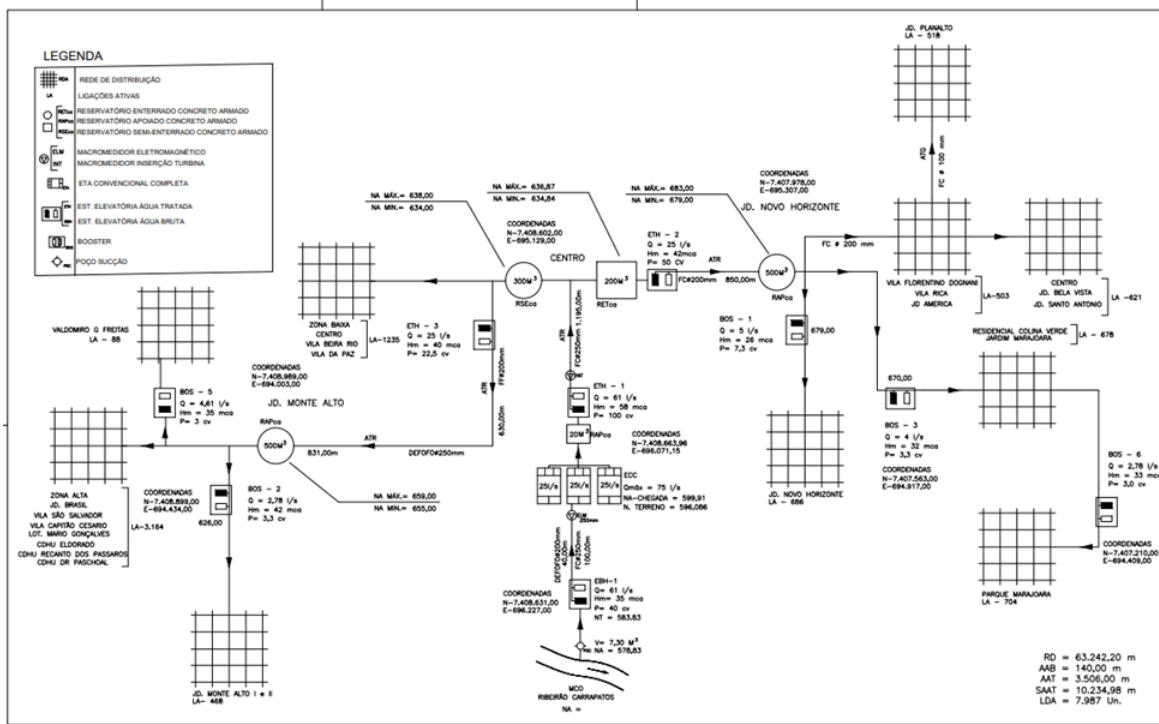
Figura 1- Croqui do sistema de abastecimento de Itaí
