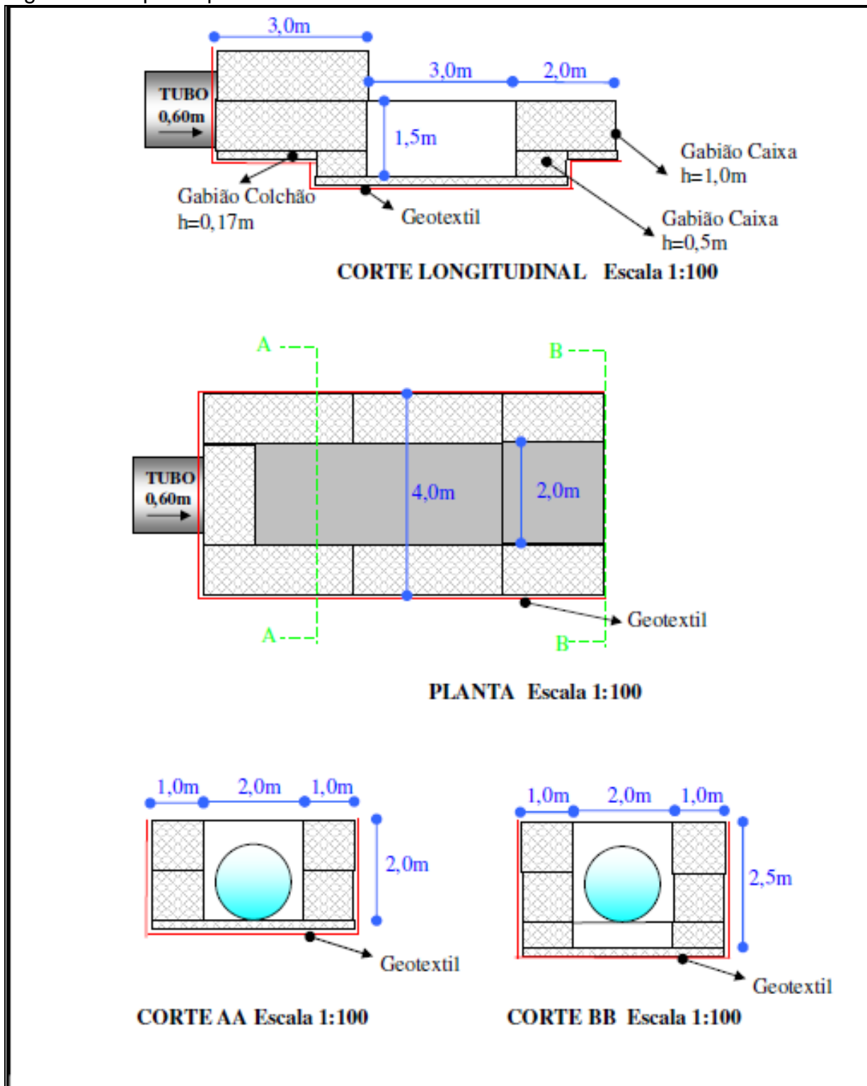
Figura – Dissipador para diâmetro de 600mm
