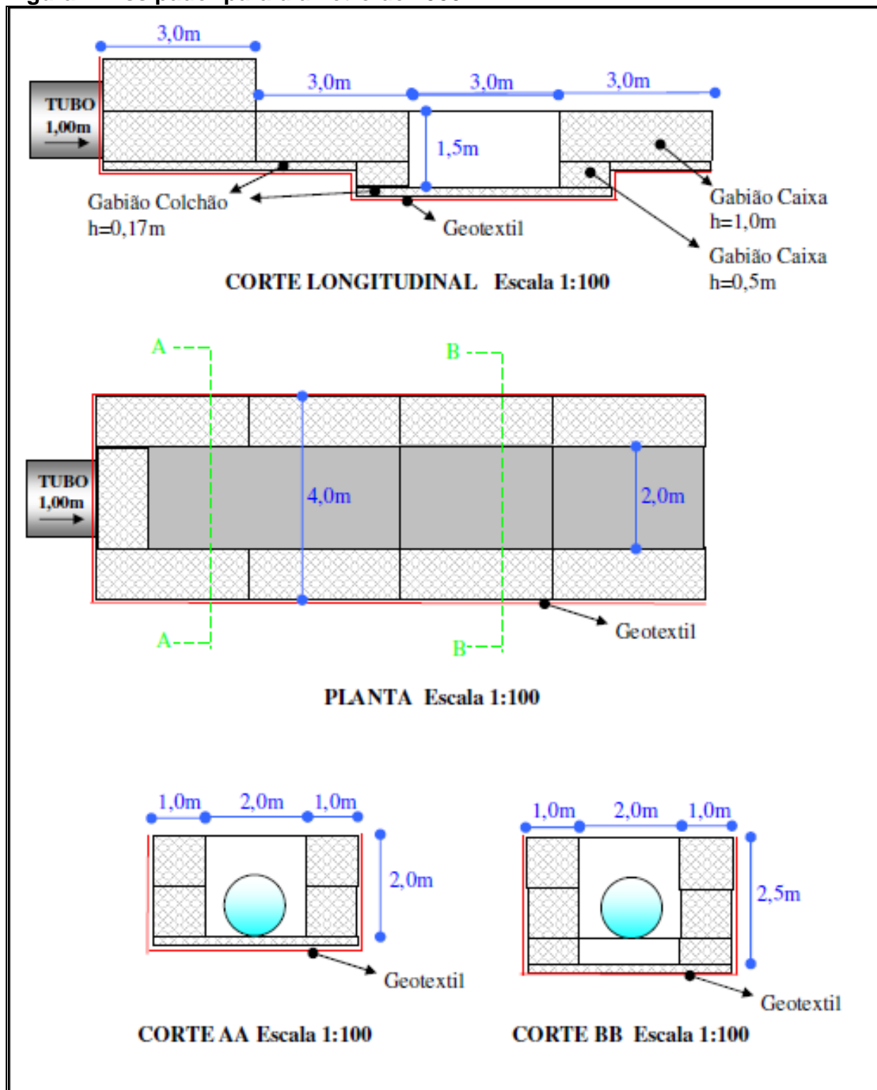
Figura – Dissipador para diâmetro de 1000mm
